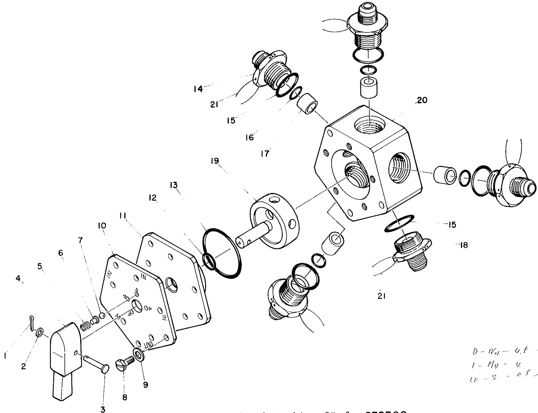
カ2-1図 ビルジ・セレクター・バルブ 232300
