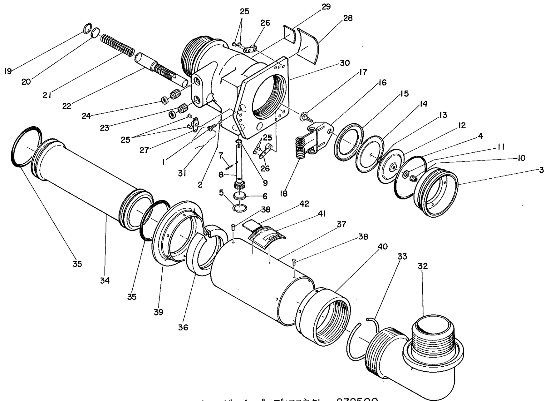
カ4-1図 ウイング・チップ・ディスクコネクタ 232500
