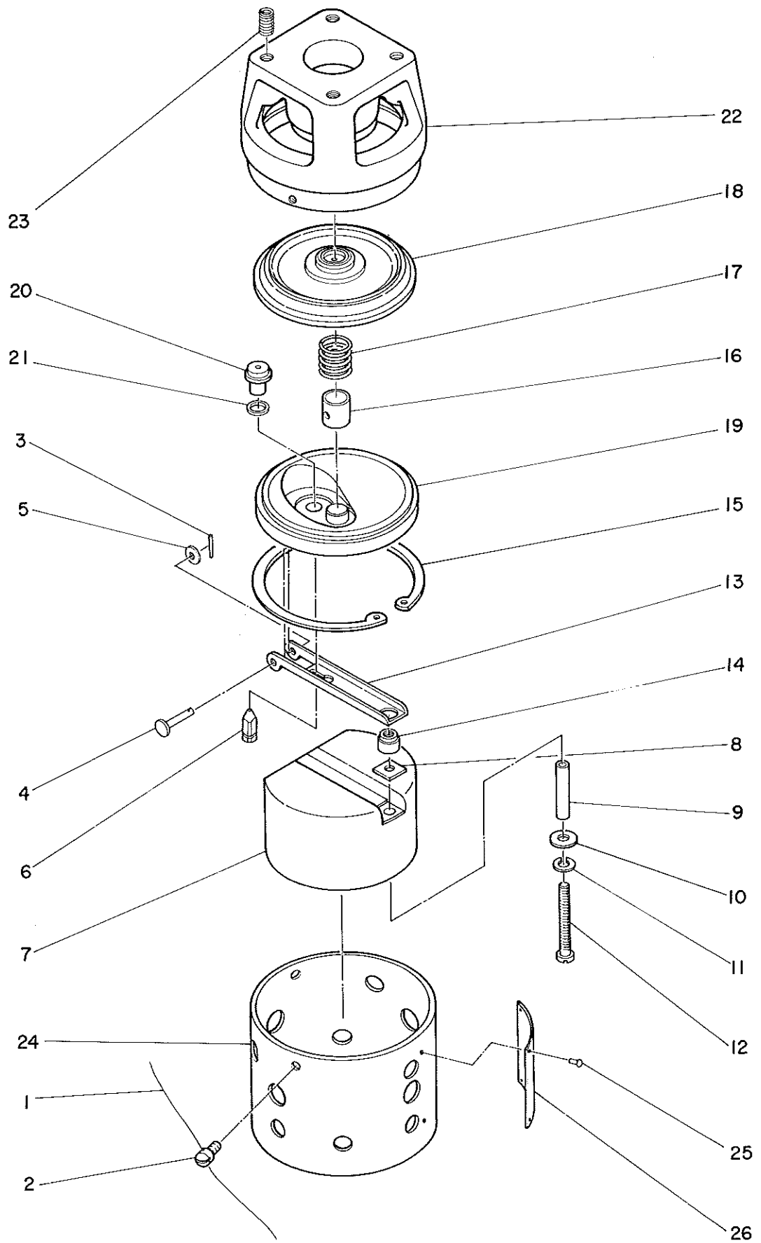
カ4-1図 フロート・バルブ 232400
