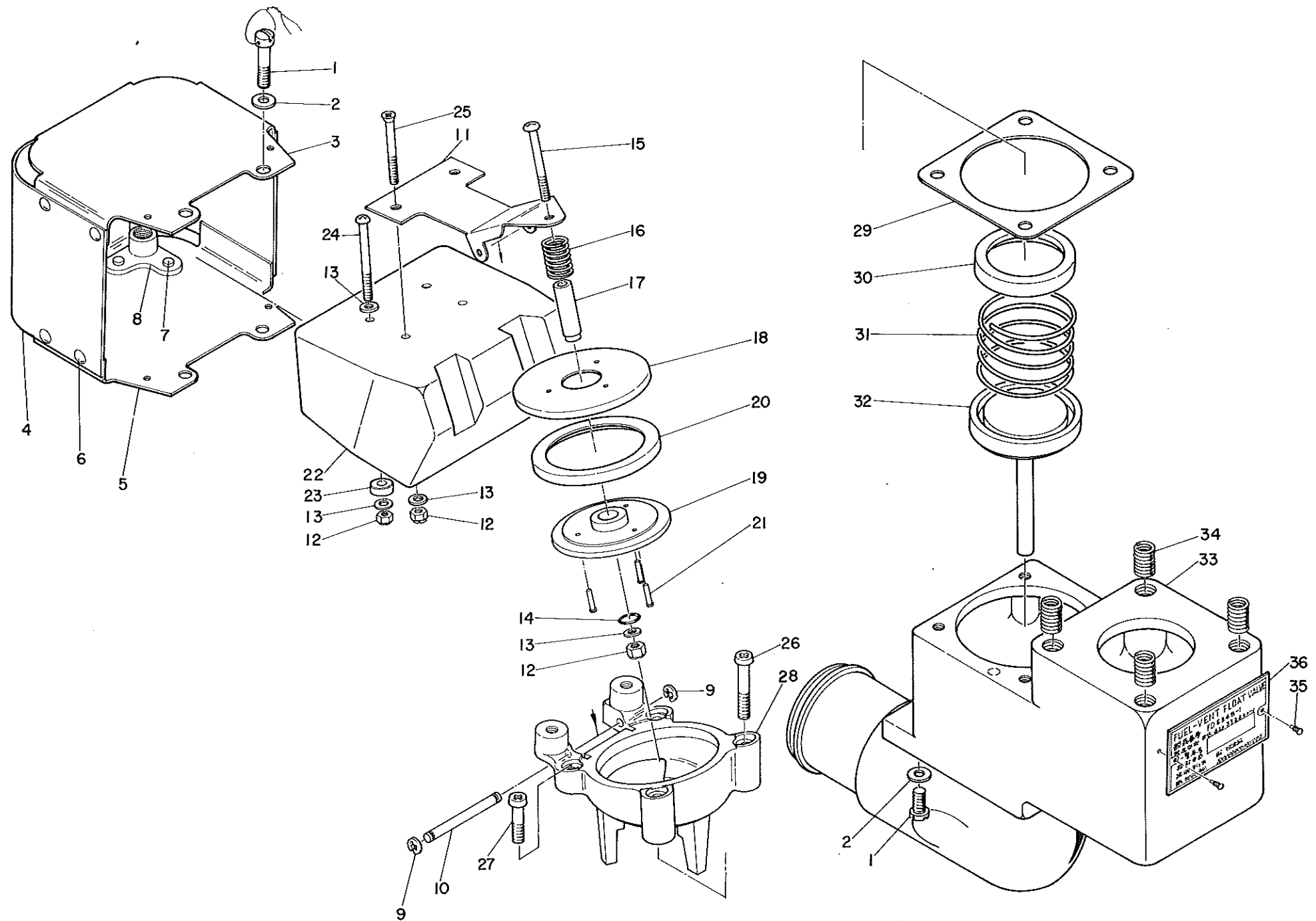
カ4-1図 フュエル・ベント・フロート・バルブ 232600
