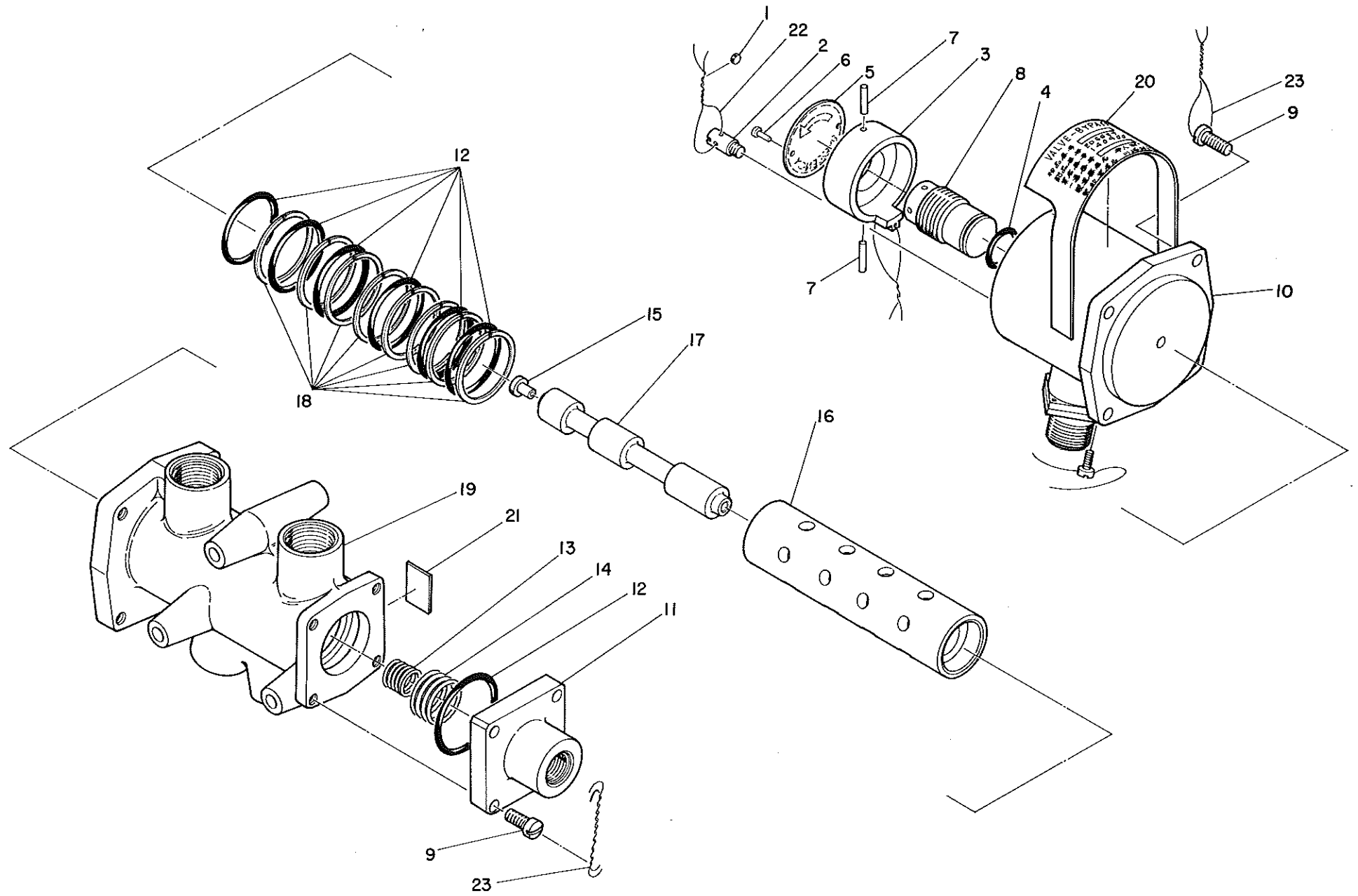
カ4-1 図 バイパス・バルブ 140900-1
