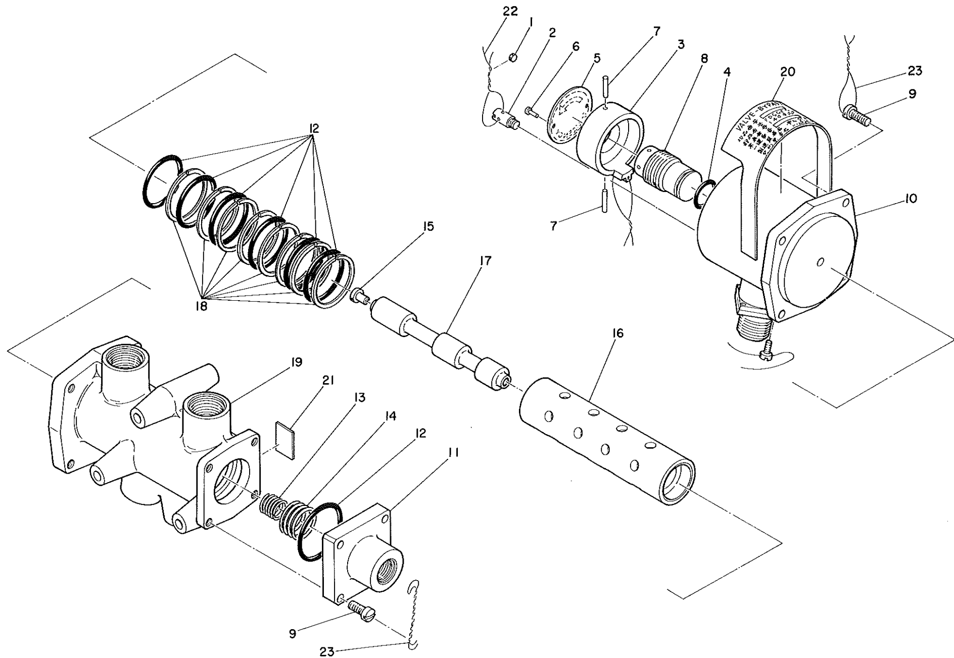
㊦4-1 ㊦ バイパス・バルブ 140900-3
