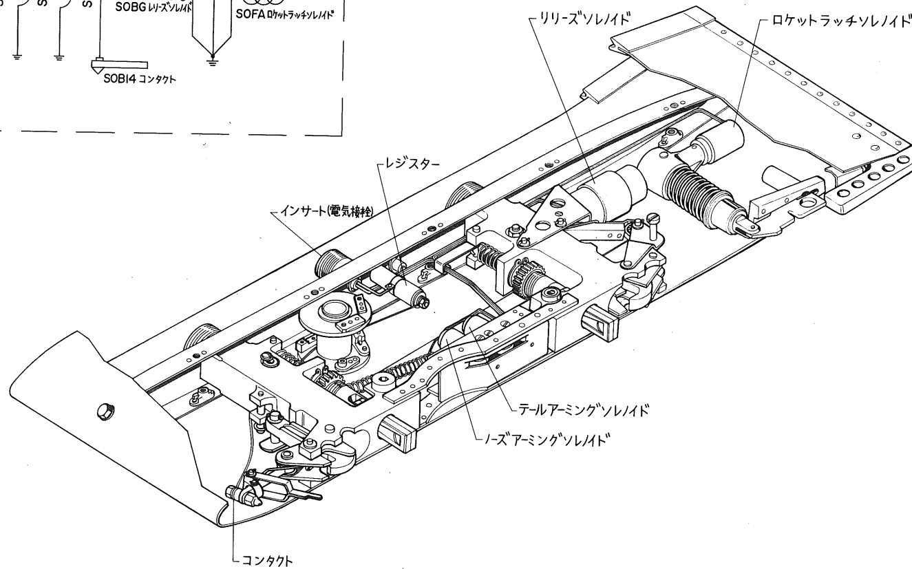
付図3 コンビネーションラック Aero14B-N 一般構造断面図及び配線図
