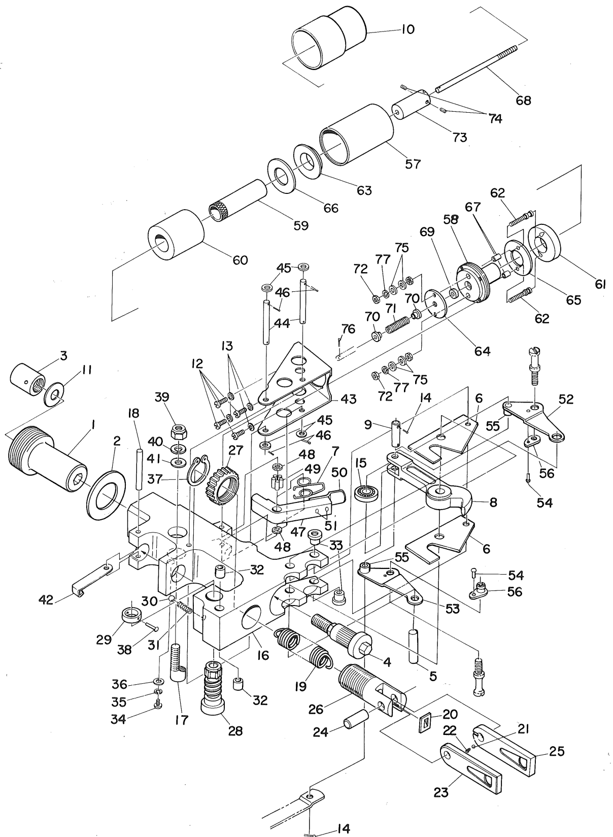
付図10 コンビネーションラック Aero 14B-N 後部サポート及び関連部品分解図
