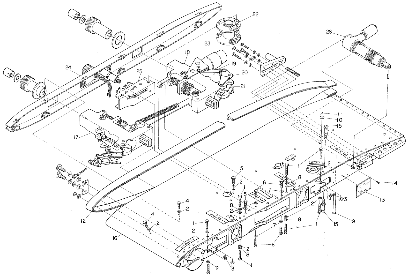
付図6 コンビネーションラック Aero14-N 大分解図
