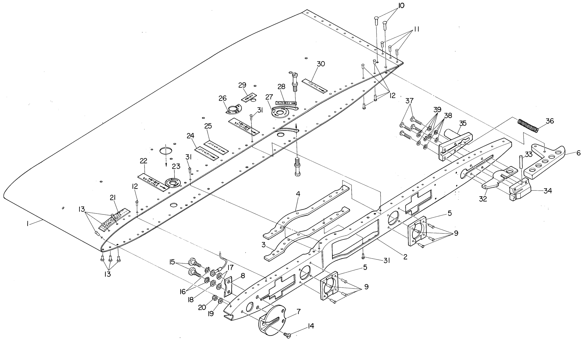
付図7 コンビネーションラック Aero14-N フェアリング組立部分解図
