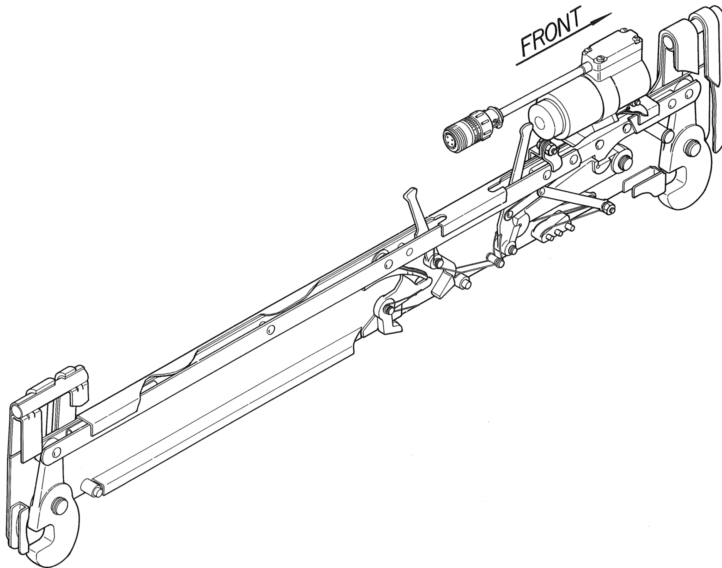
ポンプシャックル AERO 16-N 一般構造図
