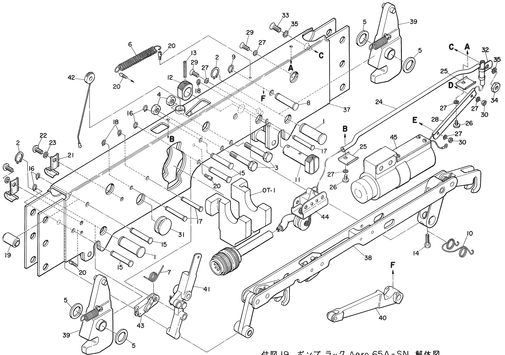
付図19 ポンプ ラック Aero 65A-SN 解体図
