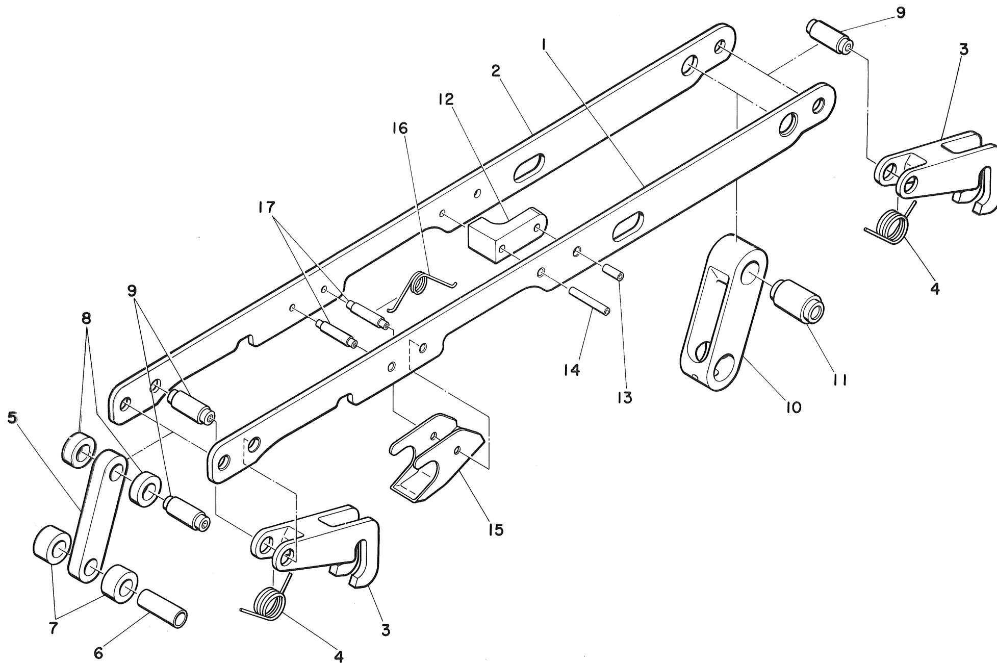
付図 21 フック タイロンケージ 組立解体図
