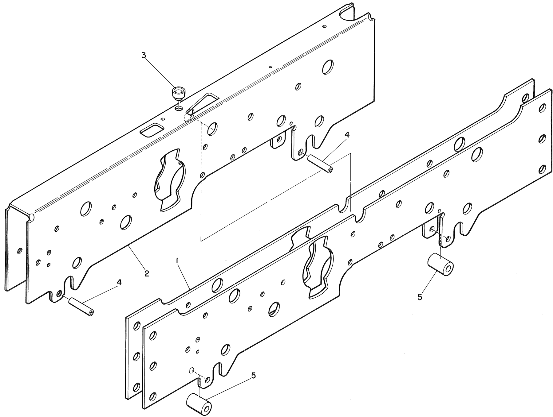
付図 20 フレーム組立解体図
