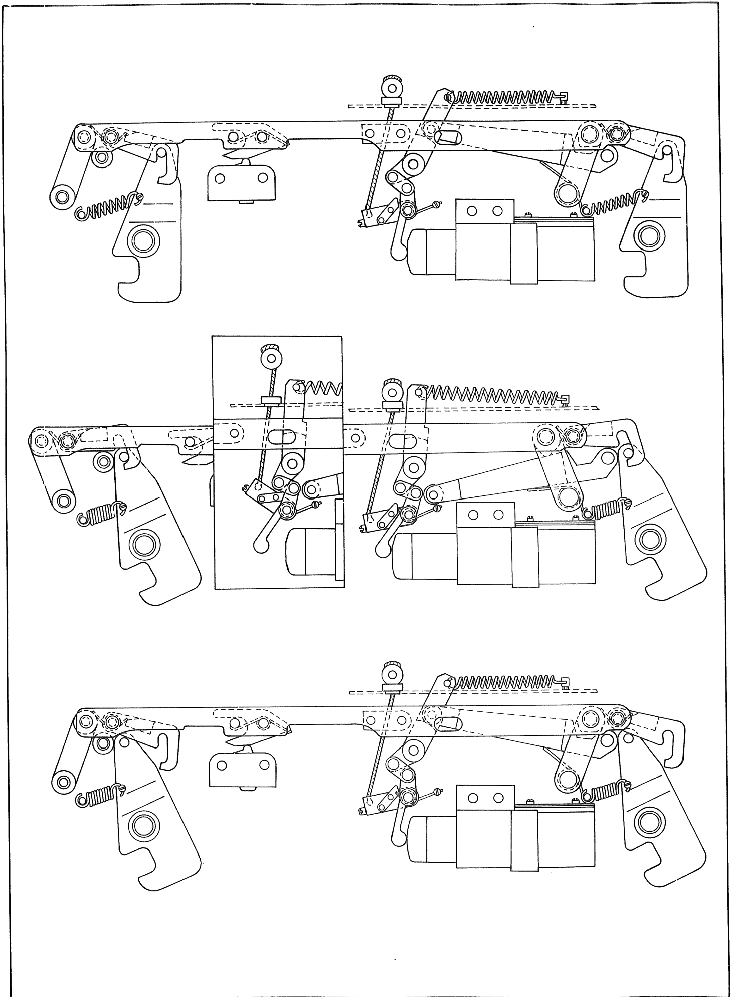
付図 8 作動機構部動作状態
